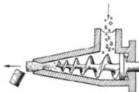
Шнековый пресс
